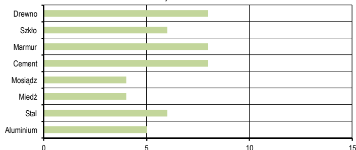
Średnia wytrzymałość na ścinanie (N/mm 2 ) różnych materiałów
