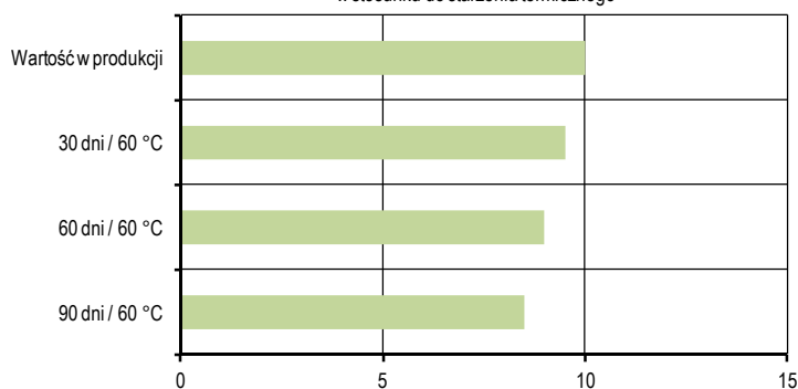
Średnia wytrzymałość na ścinanie (N/mm 2 ) w stosunku do starzenia termicznego
